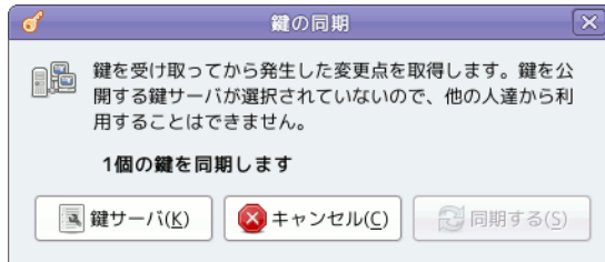
図 14 鍵の同期
